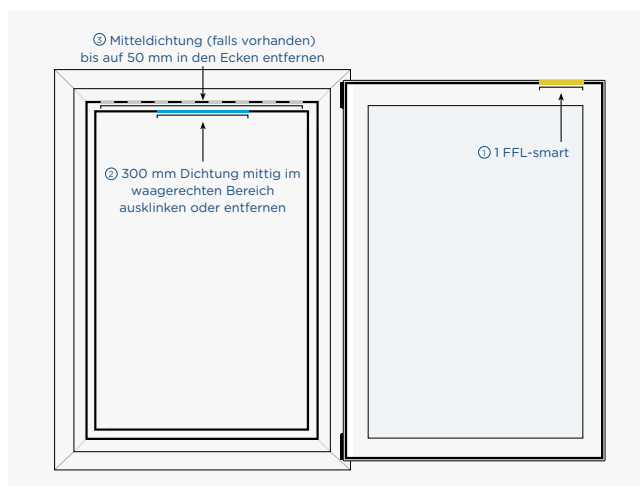
1 FFL-smart Hohe Volumenströme
