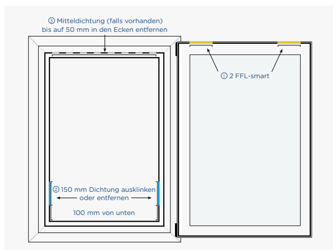
2 FFL-smart Schallschutz
