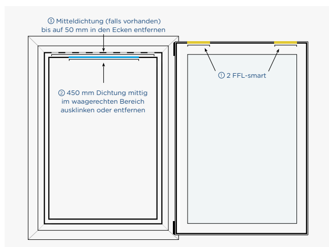
2 FFL-smart Hohe Volumenströme
