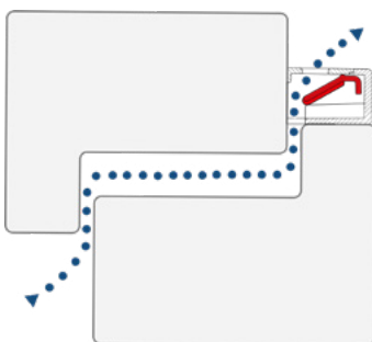
Regel-air® FFL-quick Klappe geöffnet
