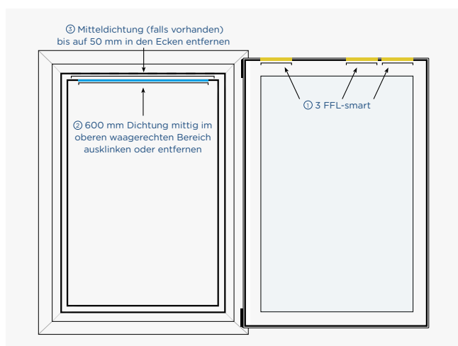
3 FFL-smart Hohe Volumenströme
