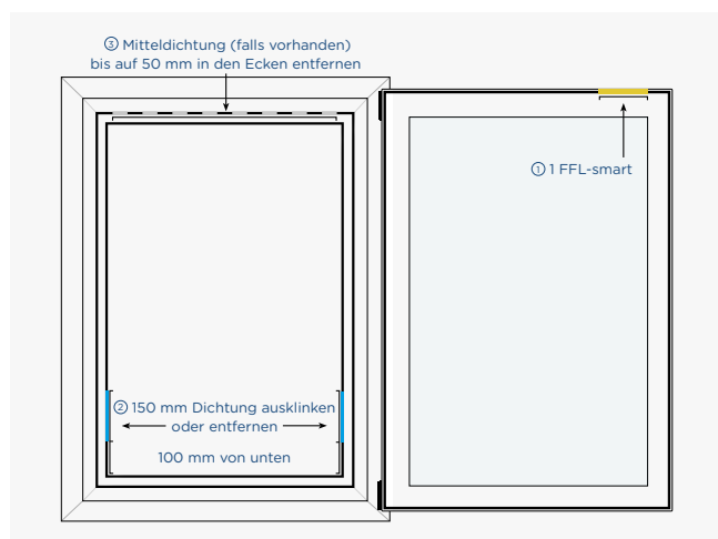
1 FFL-smart Schallschutz/Standard
