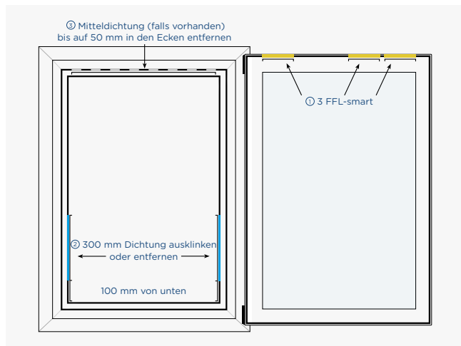
3 FFL-smart Schallschutz
