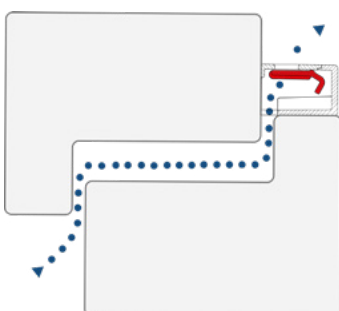
Regel-air® FFL-quick Klappe geschlossen
