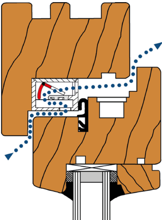
Regel-air® FFLH - Klappe geöffnet
