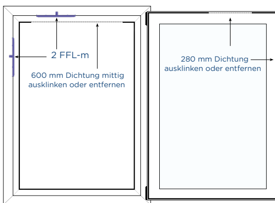
2 FFL-m – Hohe Volumenströme mit Grundlüftung Fenster mit Anschlagdichtung
