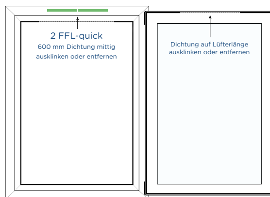
2 FFL-quick - Hohe Volumenströme Fenster mit Anschlagdichtung
