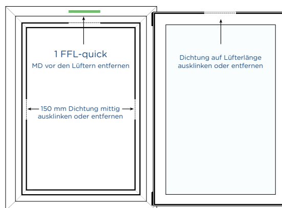
1 FFL-quick - Standard Fenster mit Mitteldichtung
