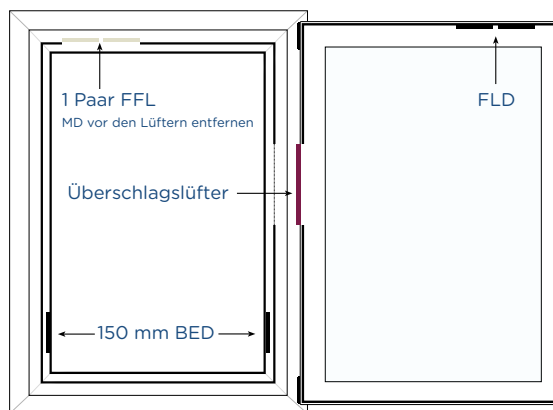
1 Paar FFL + 1 Überschlagslüfter Fenster mit Mitteldichtung
